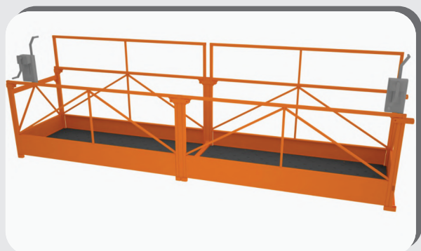
6186 Plataforma de 4 metros Peso: 238,1kg Dimensões: 910x4000x900mm Capacidade de Carga: 300kg
