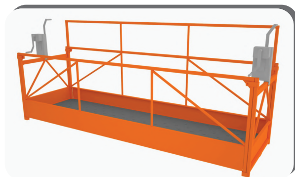
6185 Plataforma de 3 metros Peso: 183,5kg Dimensões: 910x3000x900mm Capacidade de Carga: 300kg
