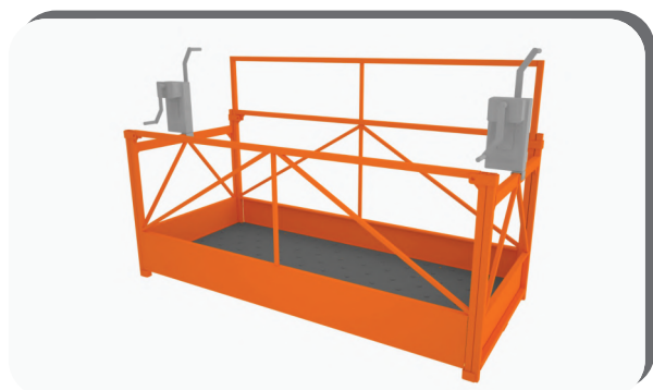
6184 Plataforma de 2 metros Peso: 148,6kg Dimensões: 910x2000x900mm Capacidade de Carga: 300kg
