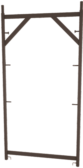
ELEMENTO VERTICAL Cód.: 6168 LAP: 1000 x 2100 x 42mm Embalagem LAP: 1000 x 2100 x 42mm Peso: 16kg
