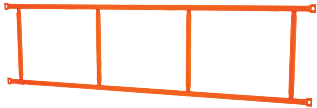
CONTRAVENTAMENTO Cód.: 2384 LAP: 2000 x 500 x 32mm Embalagem LAP: 2000 x 500 x 32mm Peso: 7,2kg
