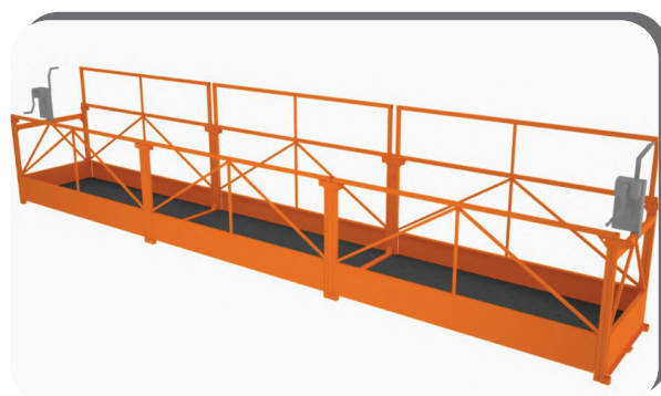
6189 Plataforma de 6 metros (3x2m) Peso: 328kg Dimensões: 910x6000x900mm Capacidade de Carga: 300kg
