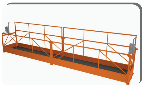
6188 Plataforma de 6 metros (2x3m) Peso: 308,2kg Dimensões: 910x6000x900mm Capacidade de Carga: 300kg
