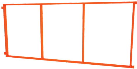
ELEMENTO HORIZONTAL Cód.: 3482 LAP: 940 x 50 x 2030mm Embalagem LAP: 940x50x2030mm Peso: 11,2kg
