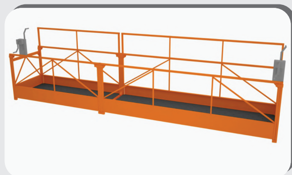
6187 Plataforma de 5 metros Peso: 273,2kg Dimensões: 910x5000x900mm Capacidade de Carga: 300kg
